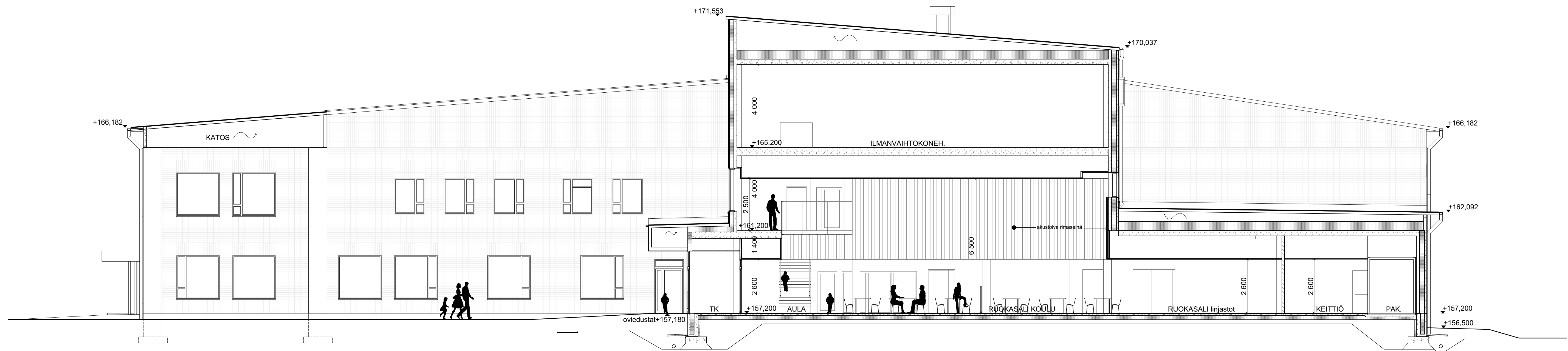
LEIKKAUS B-B 1:100
